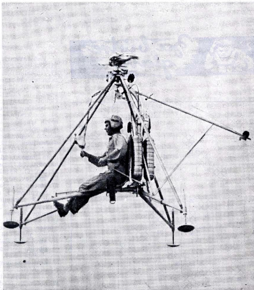
To je najnovejši model lahkega in zlozljivega helikopterja za eno osebo, kakršnega uporablja vojska ZDA. Vse potankosti o tem novem modelu so še tajnost.
