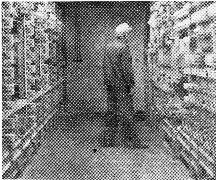
Stikalni prostor za transport surovin iz silosov na plavž
