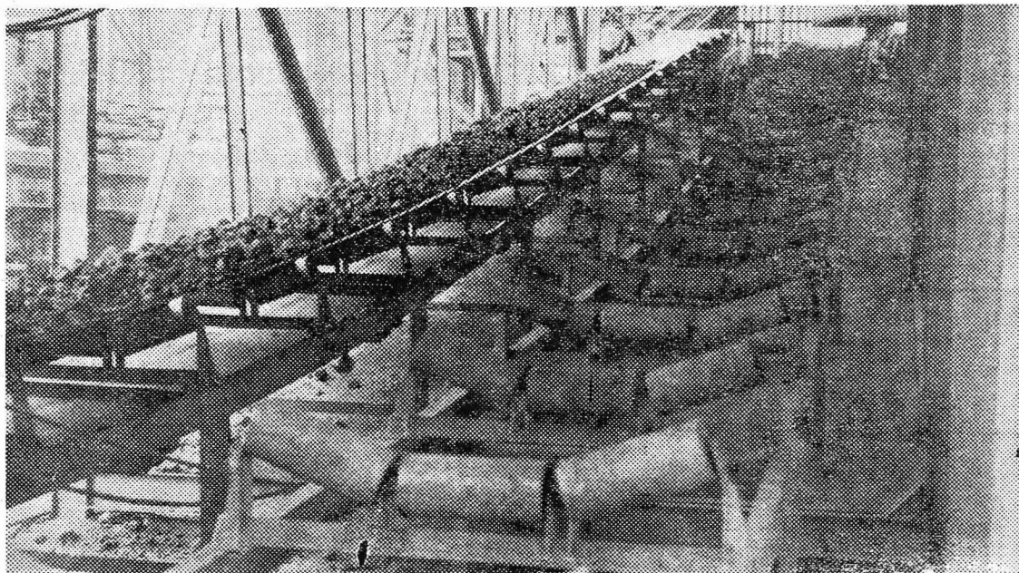
Dva trakova za dovoz surovin na plavž, od katerih eden že obratuje
