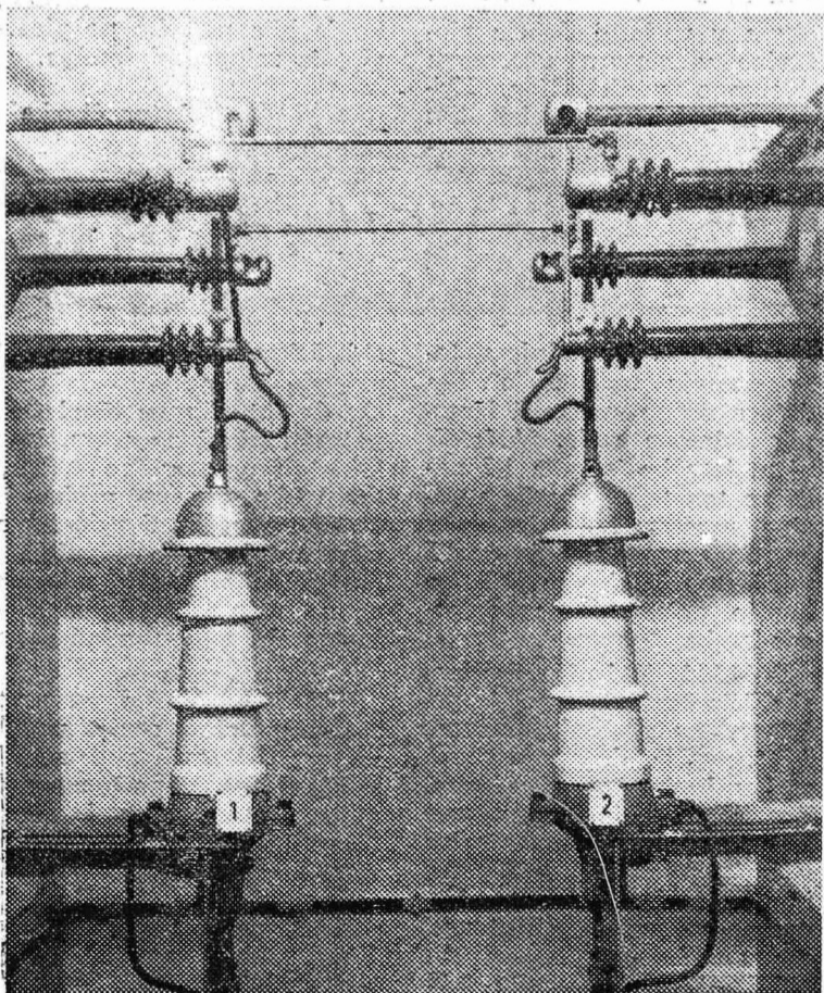
Visokonapetostni prostor za Lurgi čistilce
